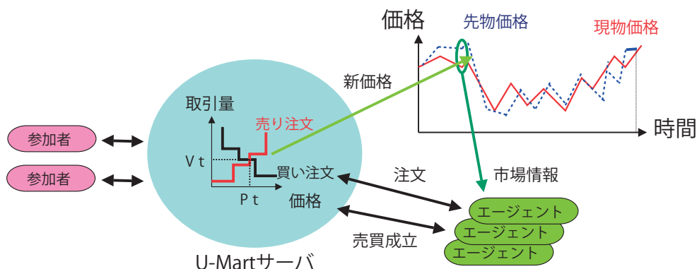
図-2 U-Martの構成
